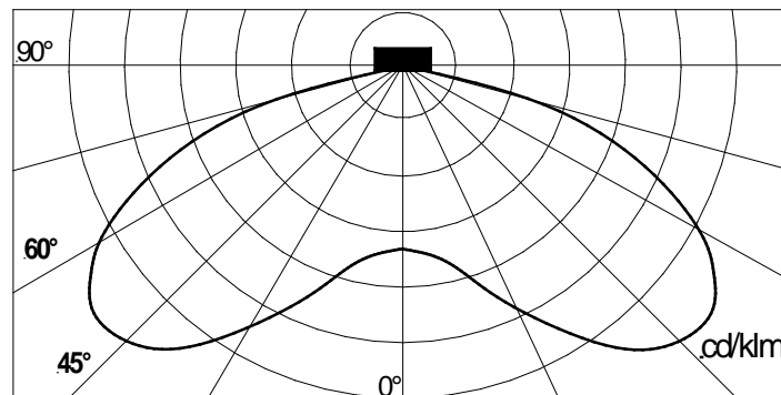
Figura 17 Ejemplo de una distribución simétrica y directa, haz amplio
